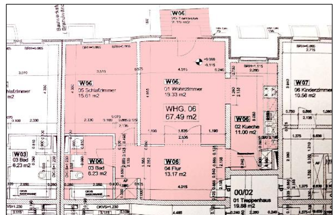
Grundriss
