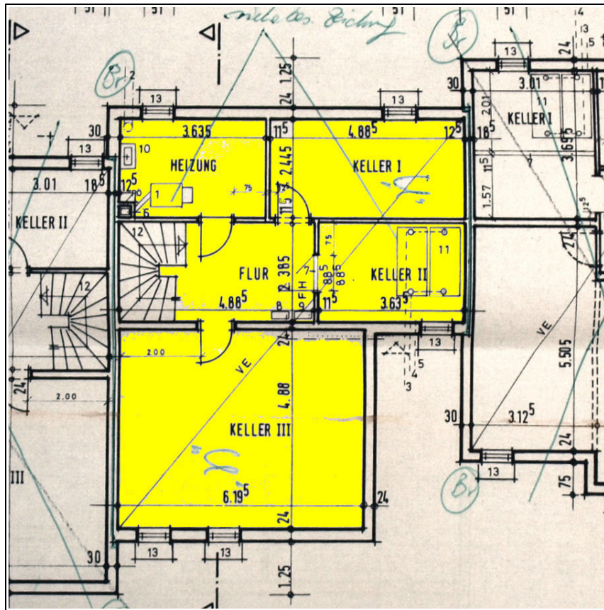
Abbildung 4: Grundriss Kellergeschoss
