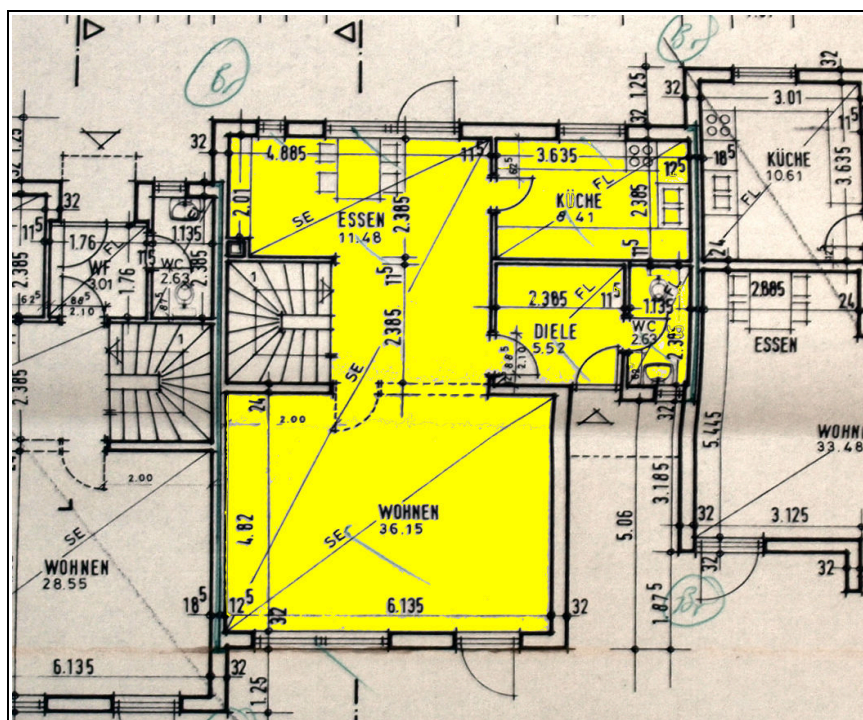
Abbildung 5: Grundriss Erdgeschoss
