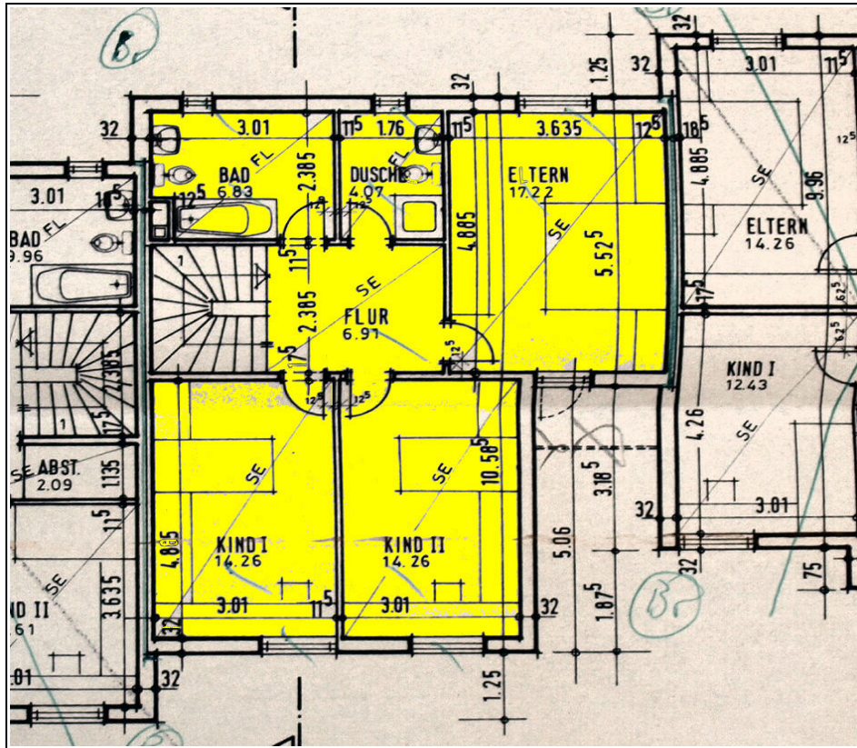
Abbildung 6: Grundriss Obergeschoss
