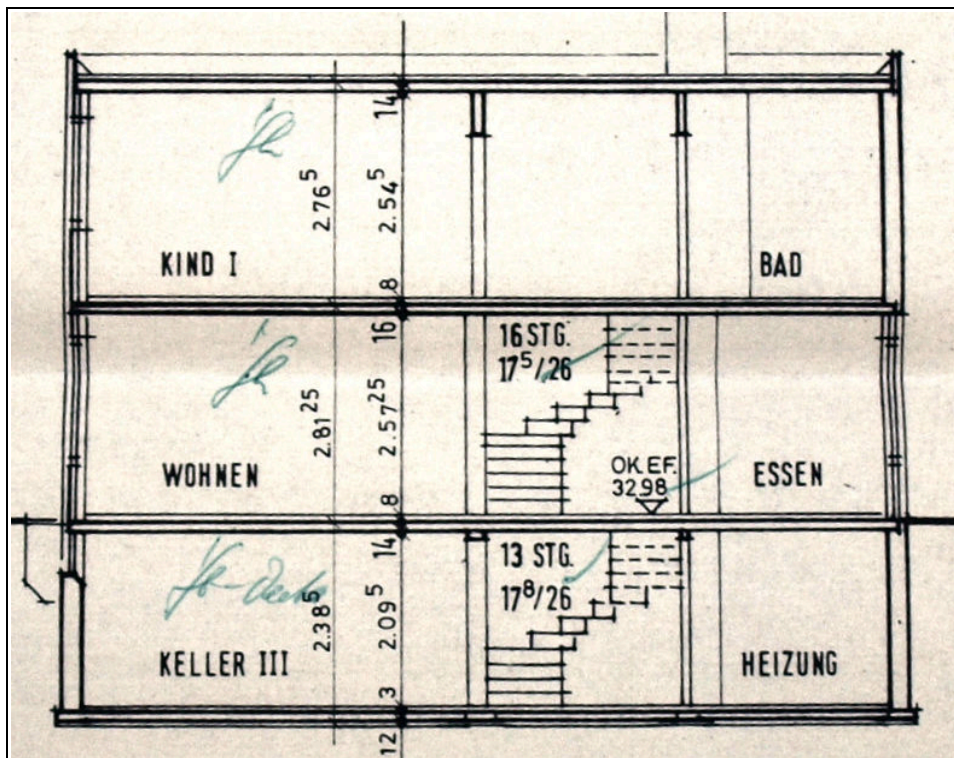
Abbildung 7: Schnittdarstellung
