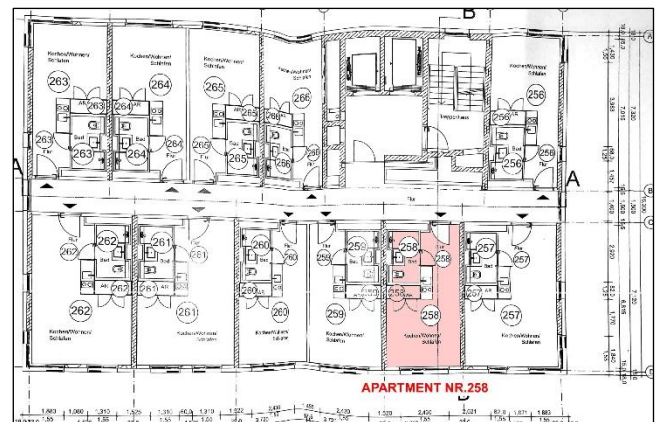
Grundriss 17. Obergeschoss
