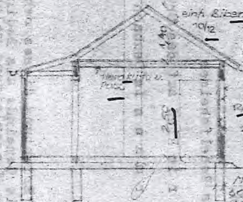
Schnitt
