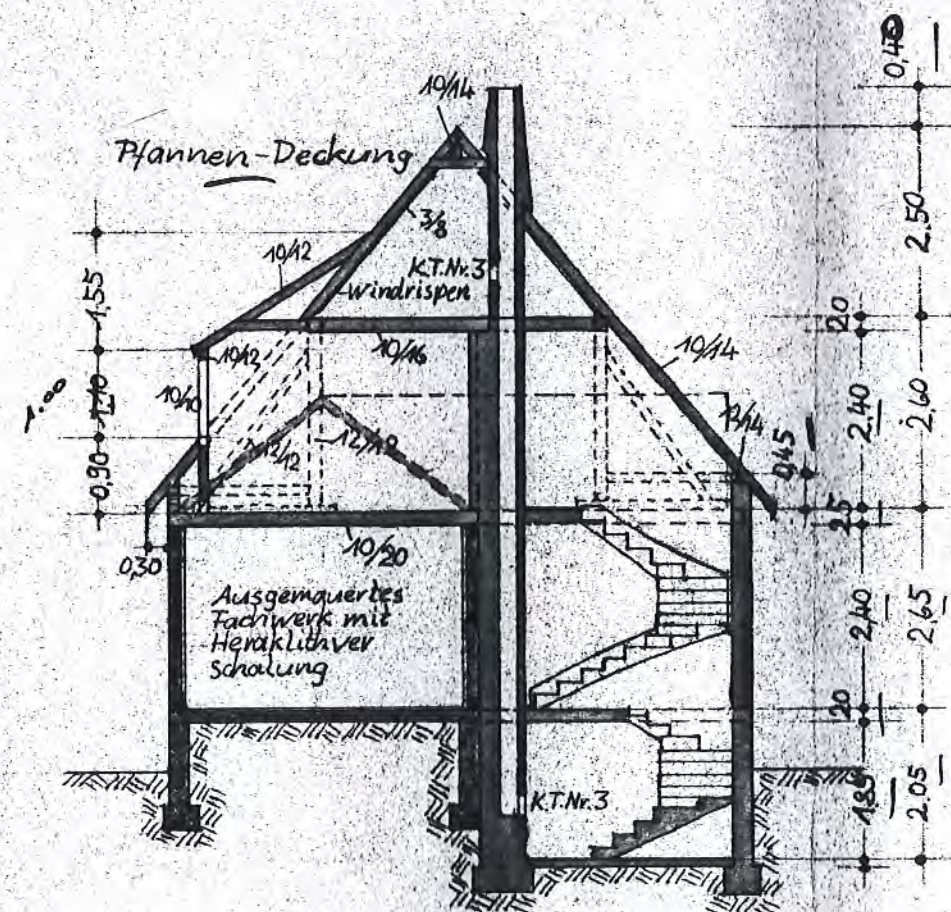
Schnitt
