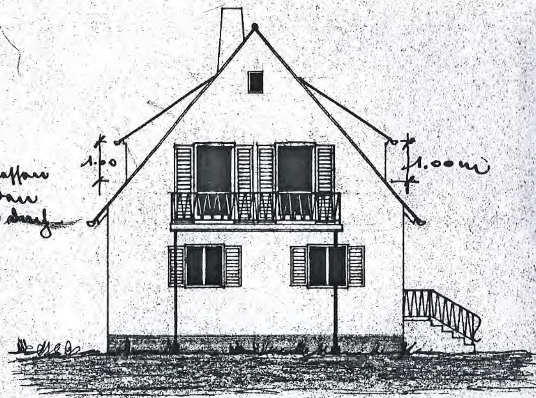
Süd-West-Seite
