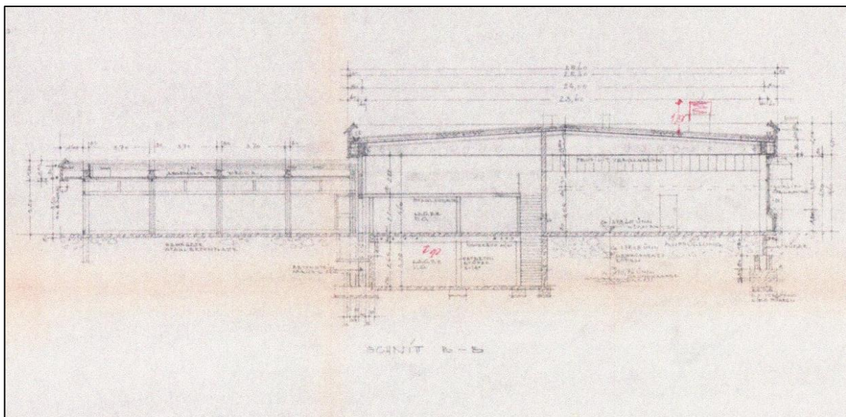
Schnitt
