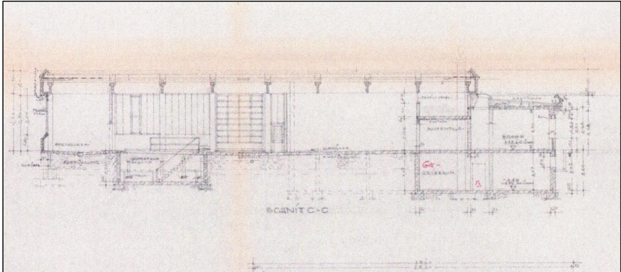
Schnitt
