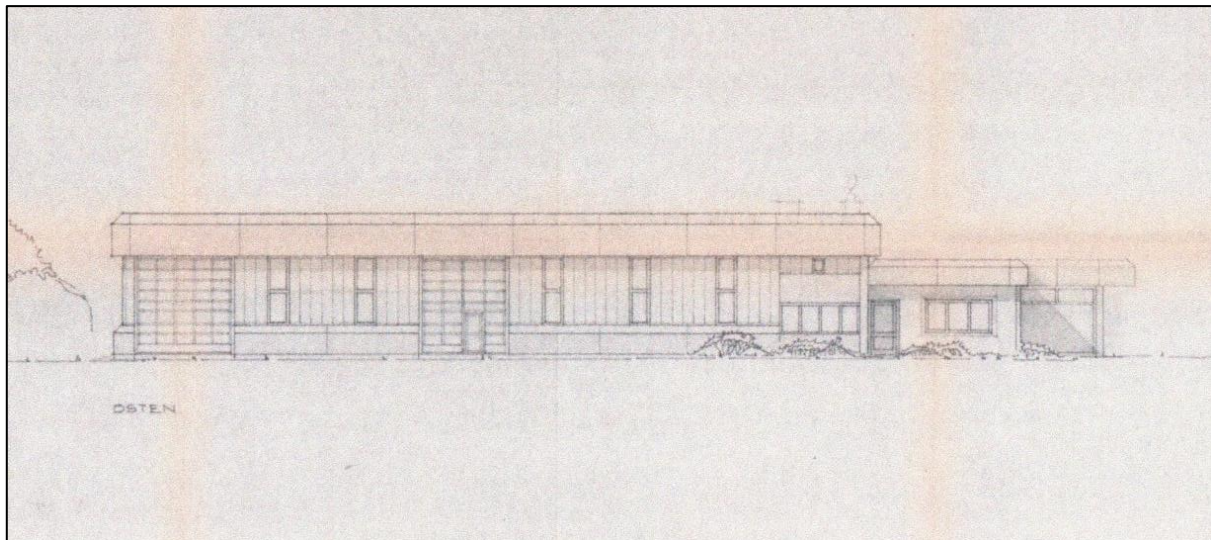
Ansicht - Osten
