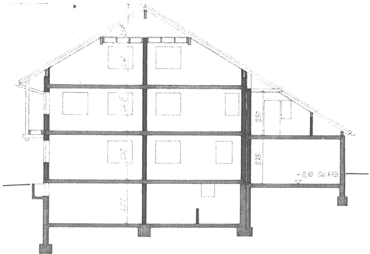
SCHNITT A-A
