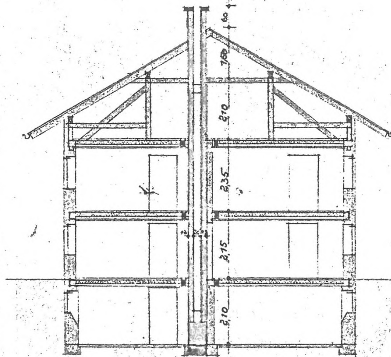
SCHNITT a-b.
