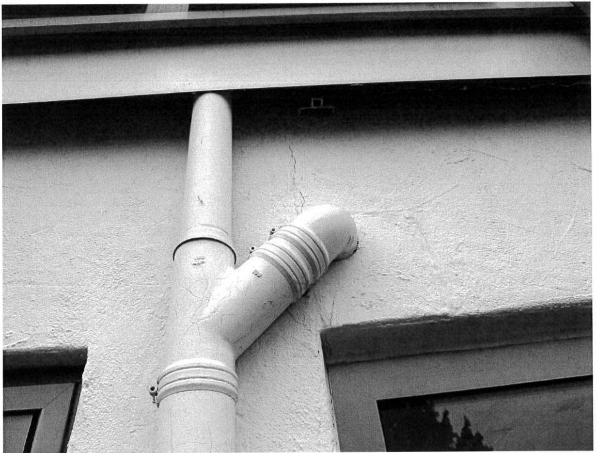
Abbildung (25) Ausstellungshalle: Fassadenriß vertikal
