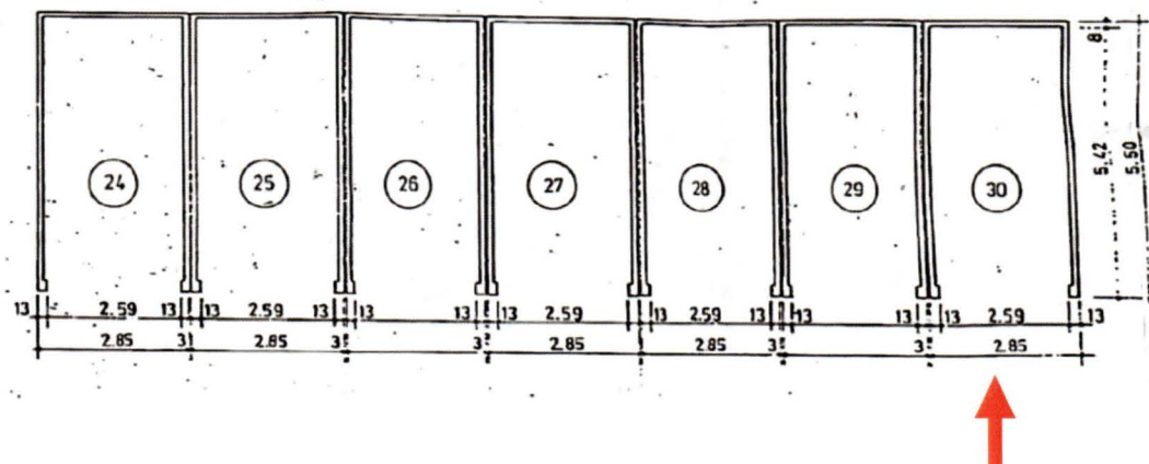
REIHENGARAGEN GRUNDRISS
