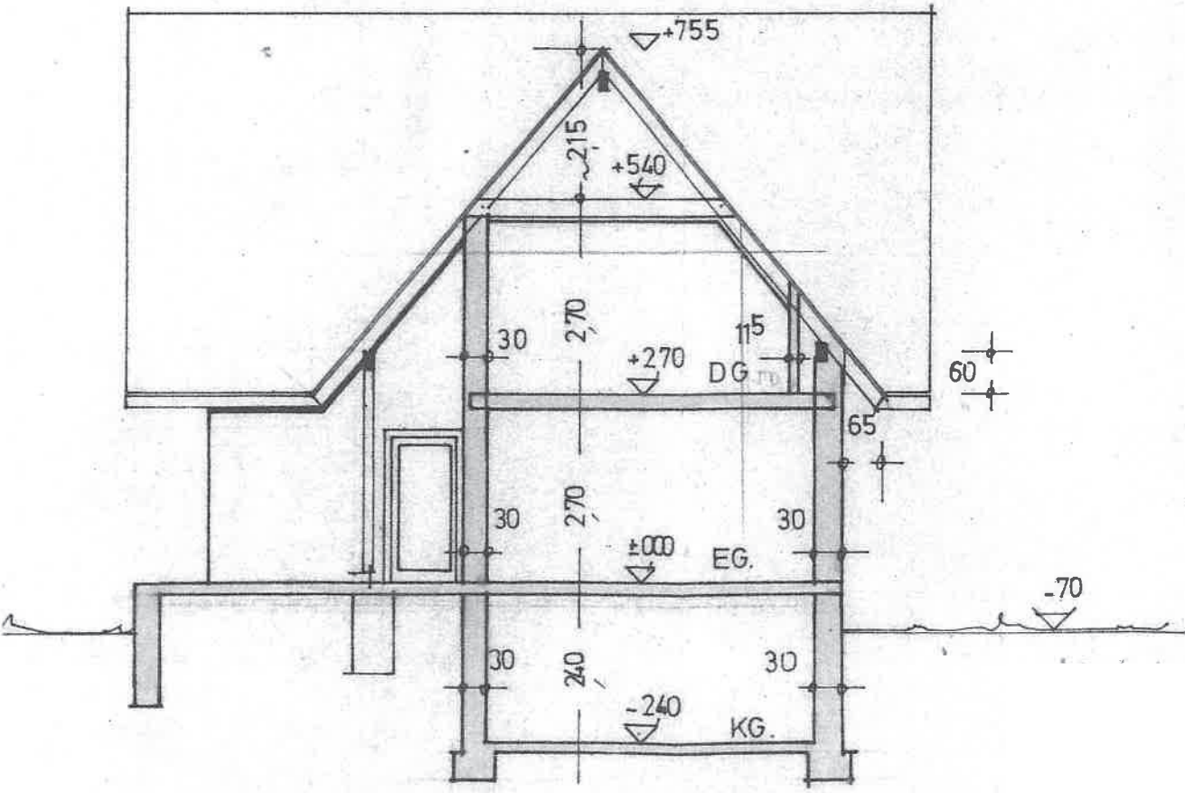
SCHNITT 3 - 4
