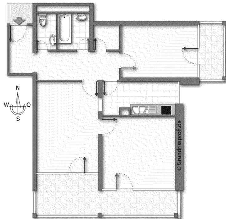
Exposé, 3. Obergeschoss, Wohnung Nr. 31, ohne Maßstab
