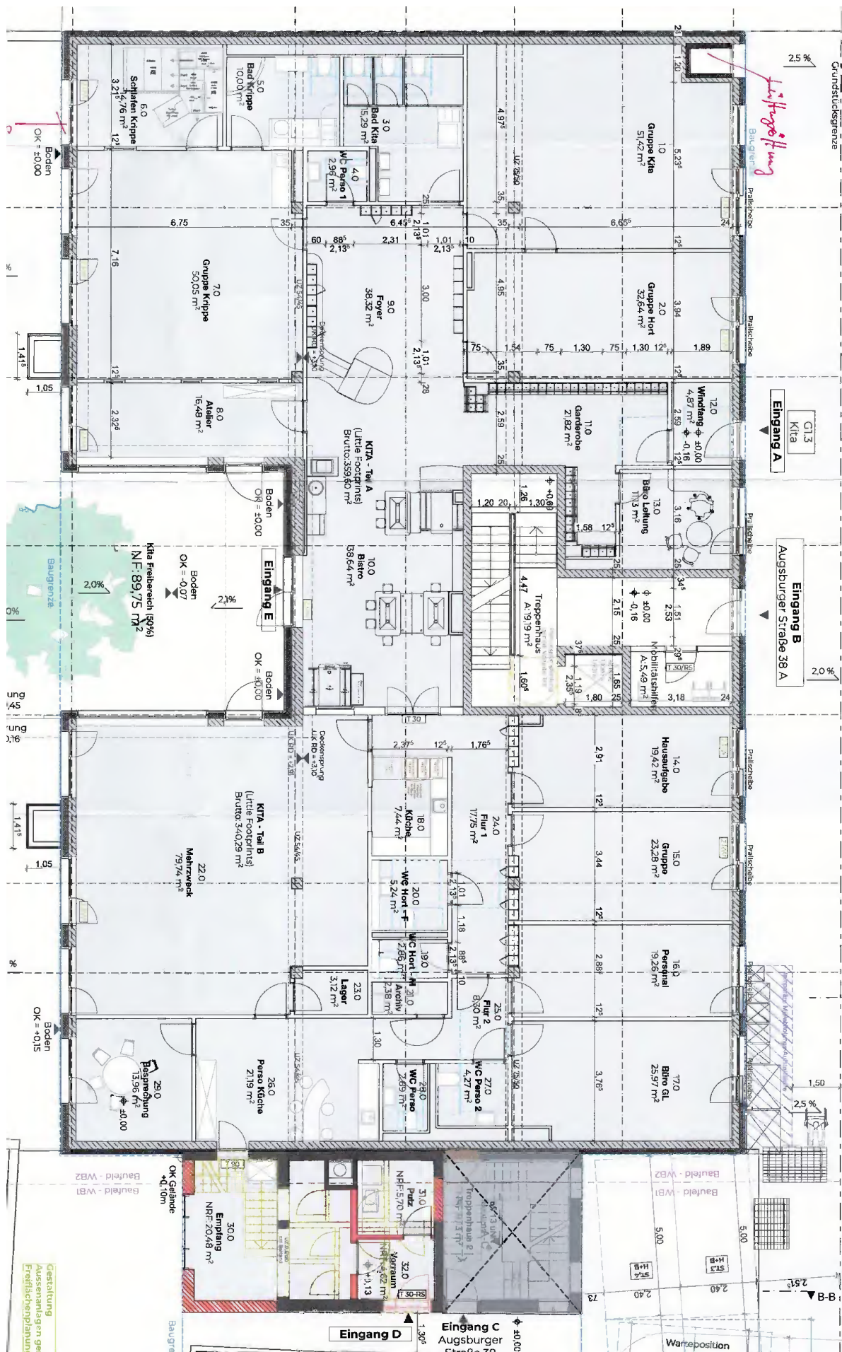
Grundriss Erdgeschoß (Planung)
