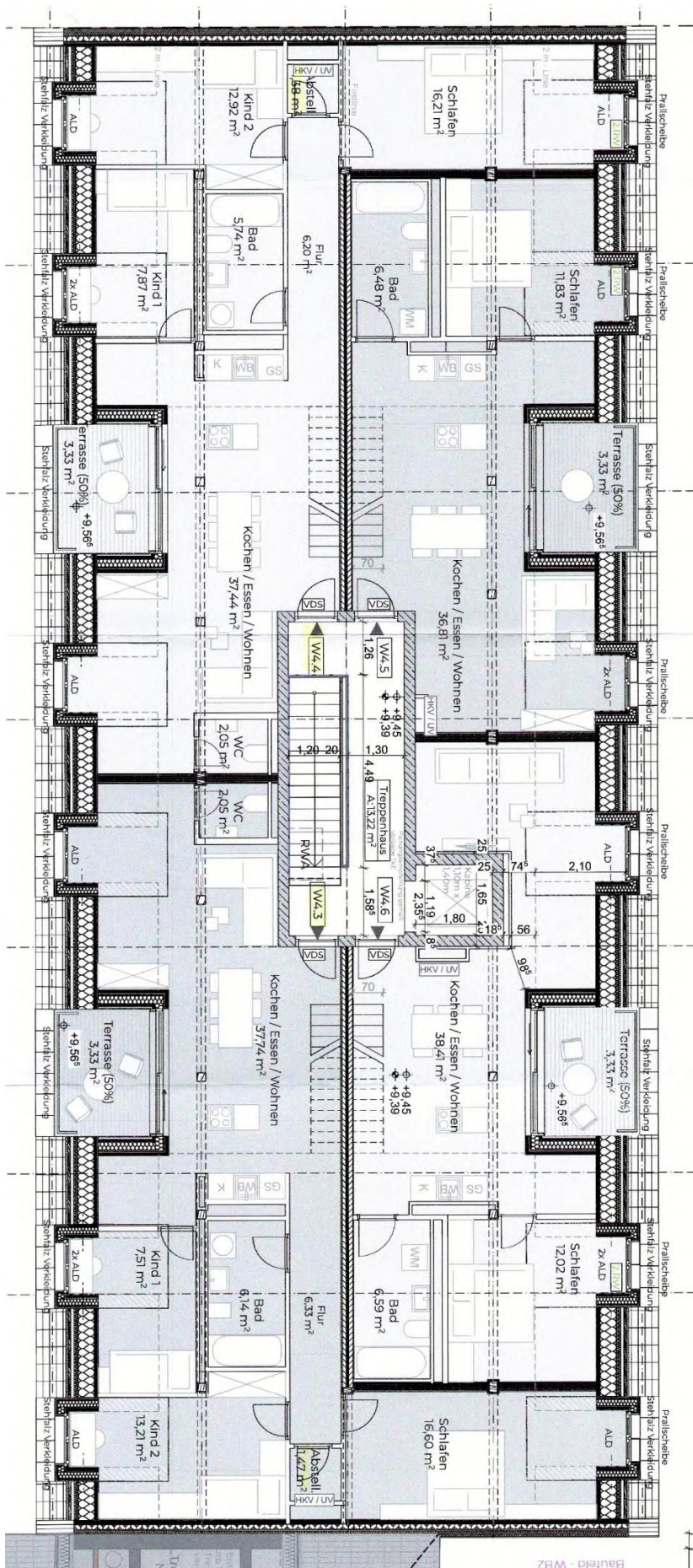
Grundriss Dachgeschoß (Planung)
