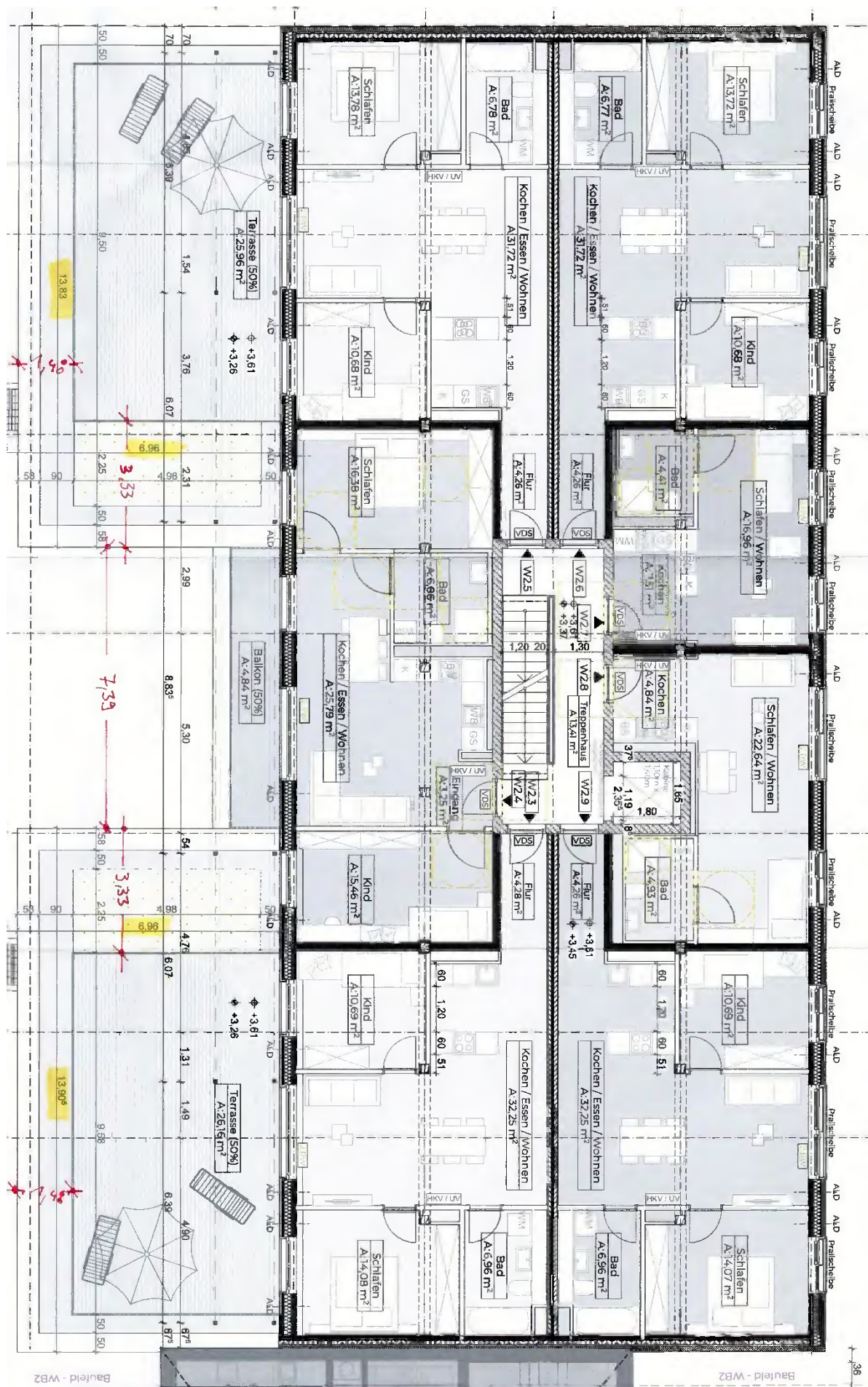
Grundriss 1. Obergeschoß (Planung)
