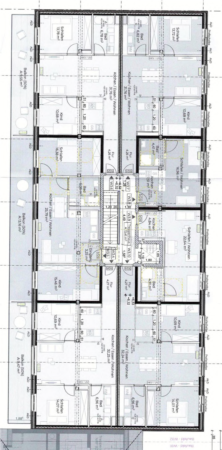
Grundriss 2. Obergeschoß (Planung)
