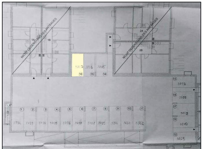
Grundriss Tiefgarage
