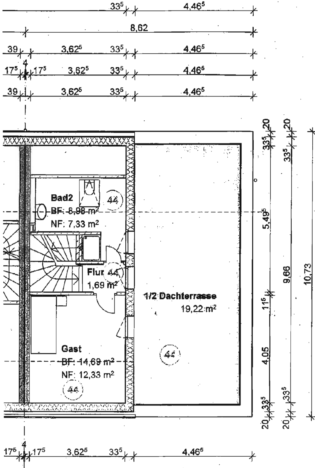
Grundriss Dachgeschoss (Ausschnitt Aufteilungsplan)
