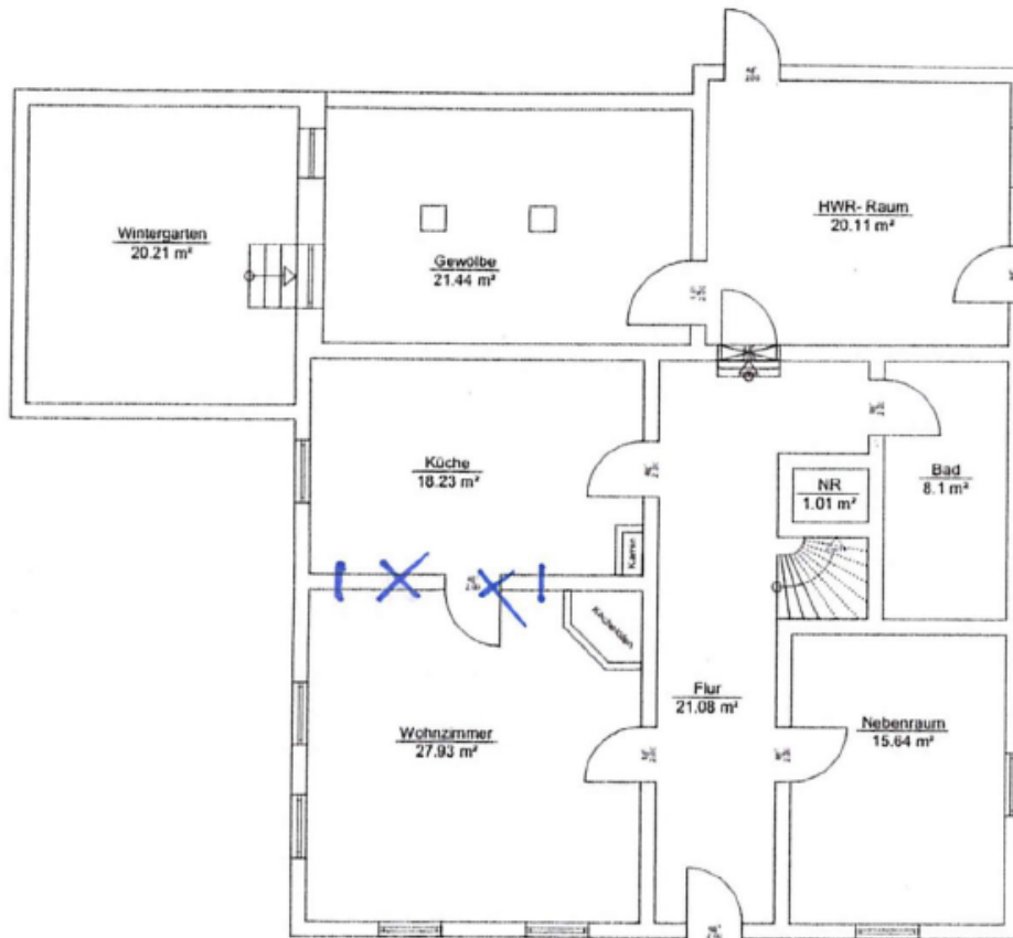
Grundriss EG
