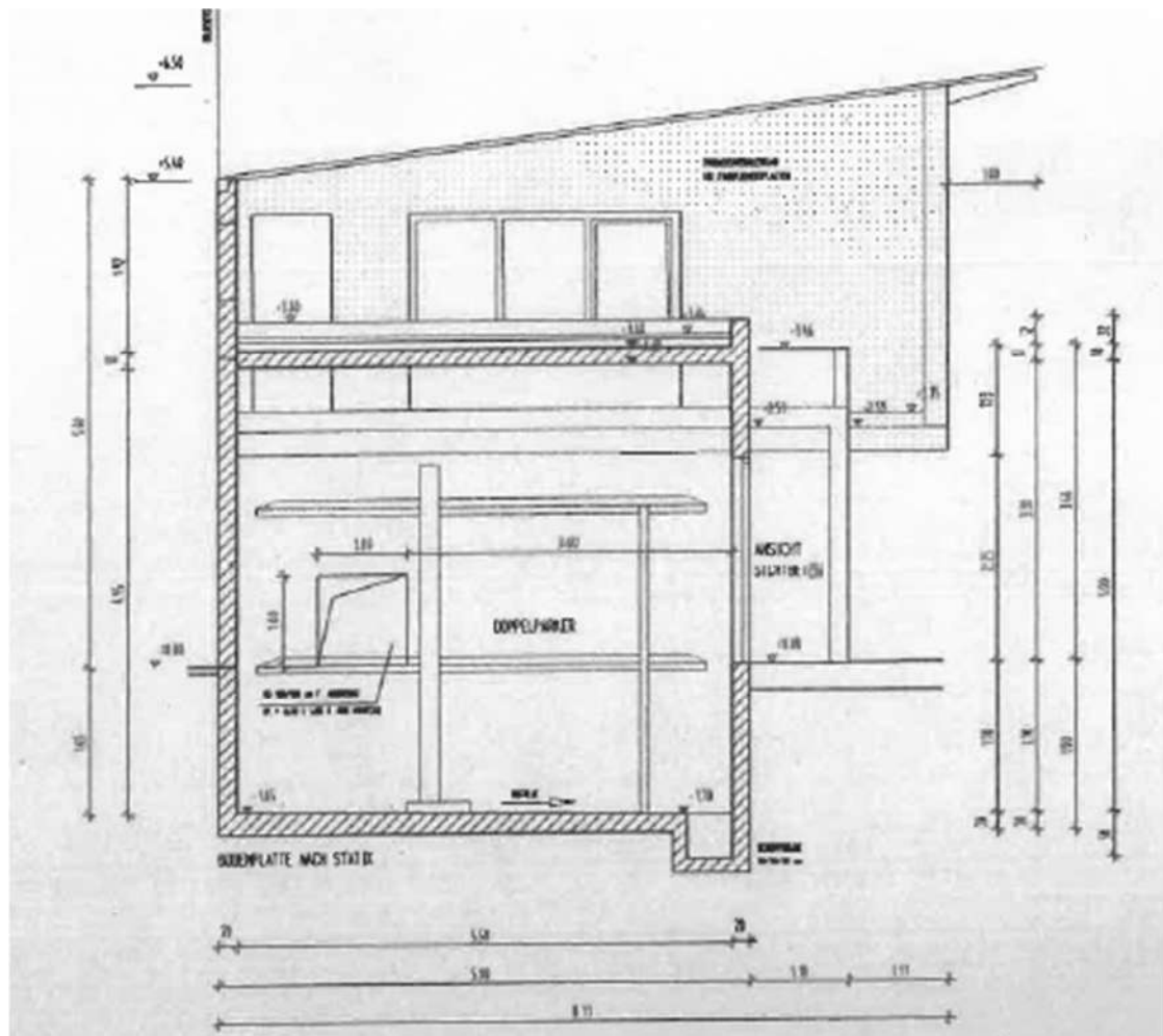
Schnitt (ohne Maßstab)
