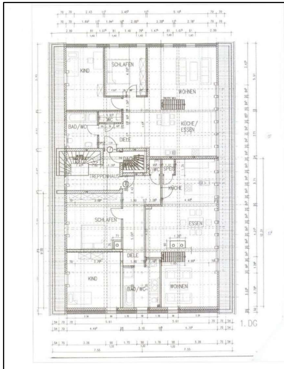
Grundriss – Dachgeschoss
