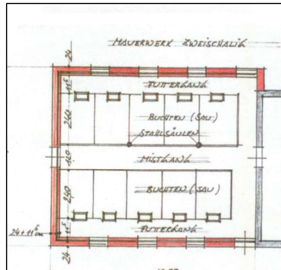
Grundriss
