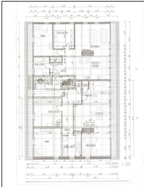
Grundriss – Dachgeschoss
