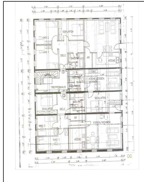
Grundriss - Obergeschoss
