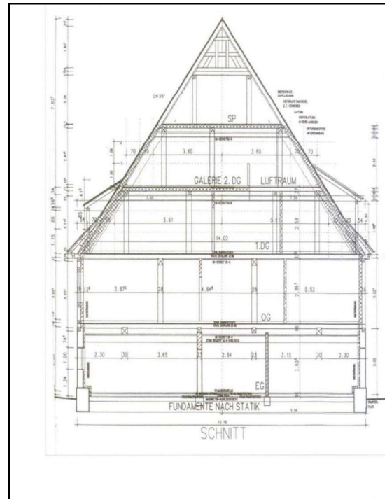
Schnitt
