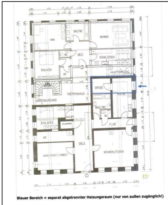
Grundriss – Erdgeschoss
