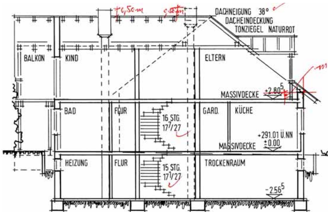
Schnitt
