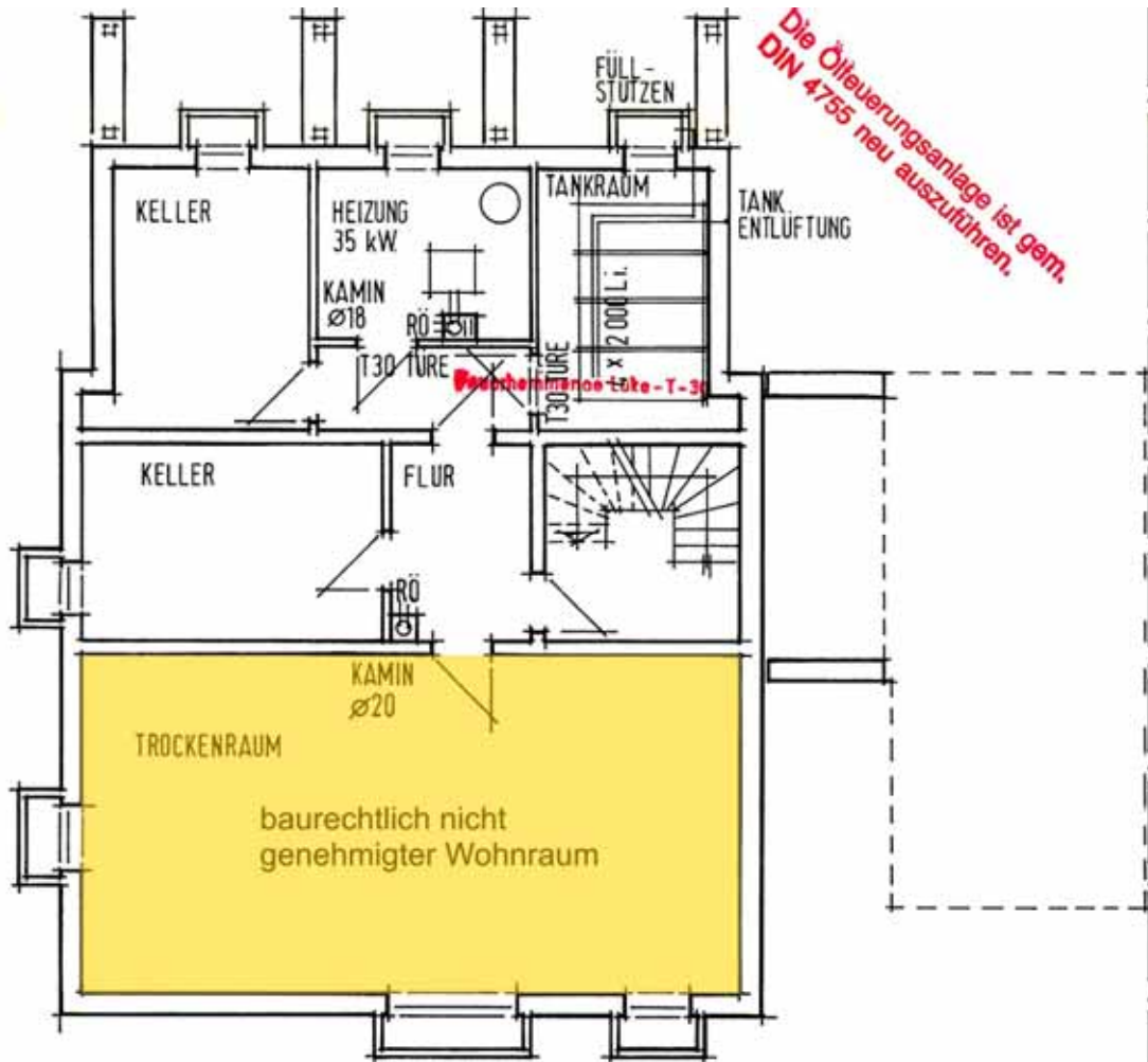
Kellergeschoss
