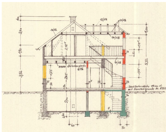
Best. Einfamilienhaus - Querschnitt
