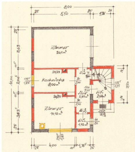
Best. Einfamilienhaus - Grundriss Erdgeschoss
