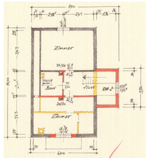
Best. Einfamilienhaus - Grundriss Obergeschoss
