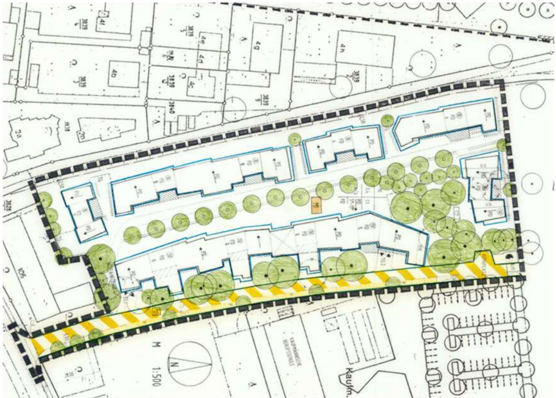
Ausschnitt aus dem Bebauungsplan (ohne Maßstab)
