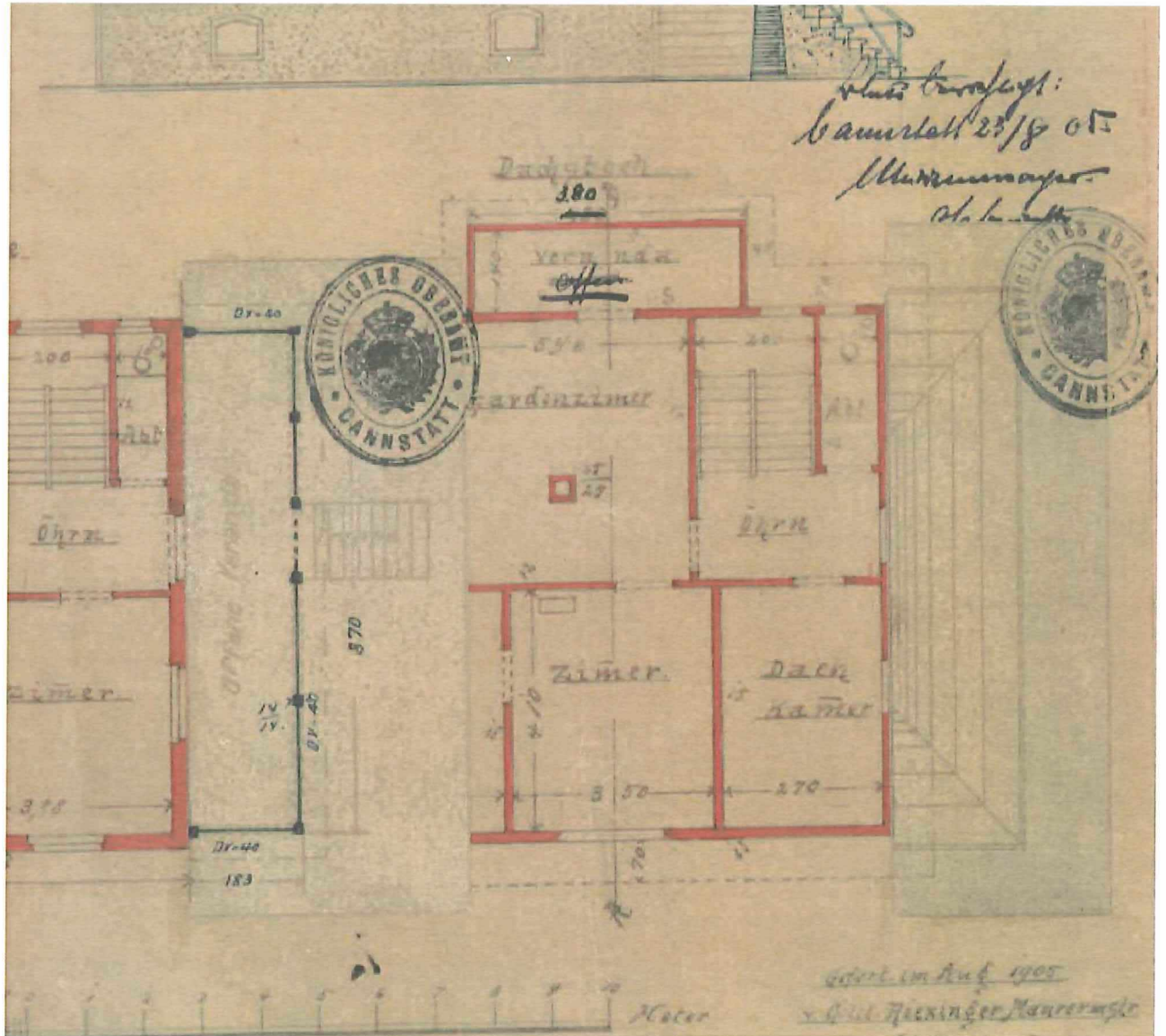
Anlage 2 b – Grundriss DG nach genehmigten Planunterlagen von 1905 / Ausschnitt
