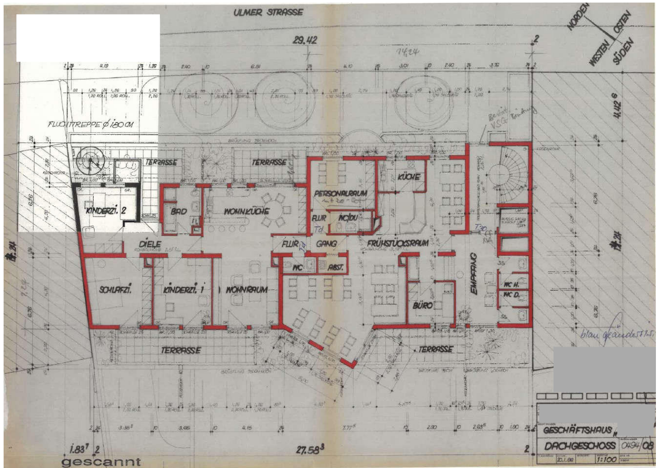
Anlage 2 g –Grundriss DG nach genehmigten Planunterlagen
