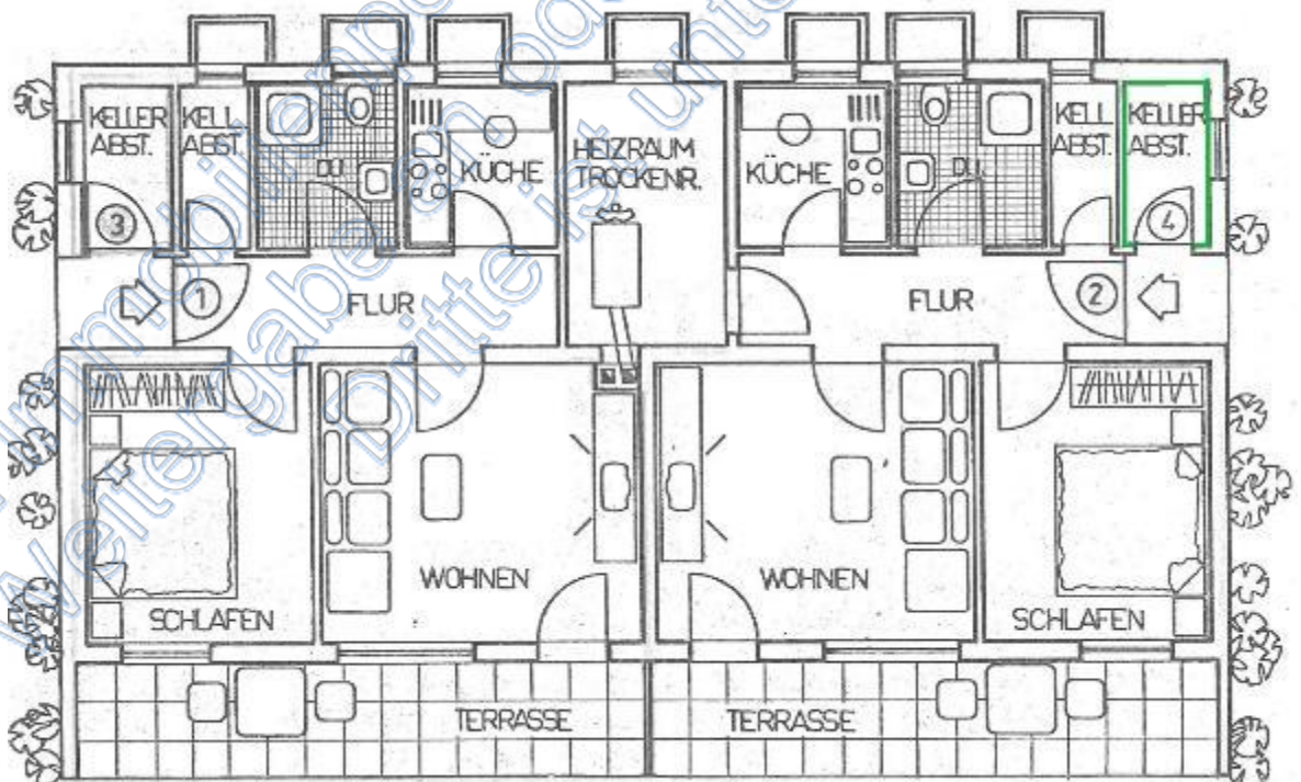
Grundriss EG, Abstellraum 4
