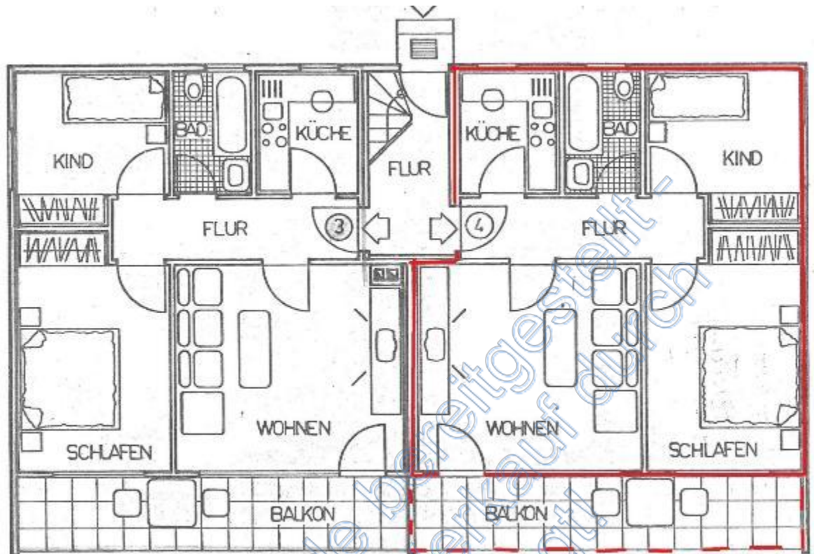
Grundriss OG, ETW 4
