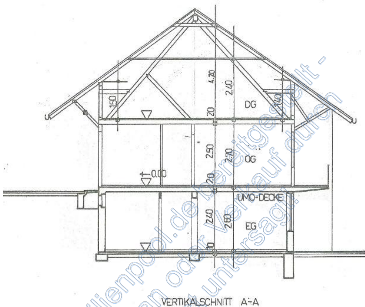
Schnitt
