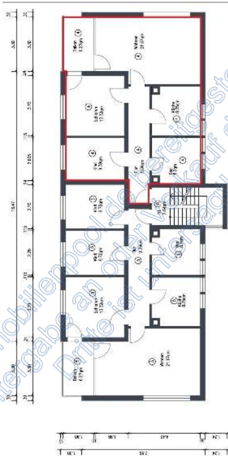
Grundriss Obergeschoss mit rot markiertem Sonder Eigentum Nr. 4 (aus Teilungserklärung)
