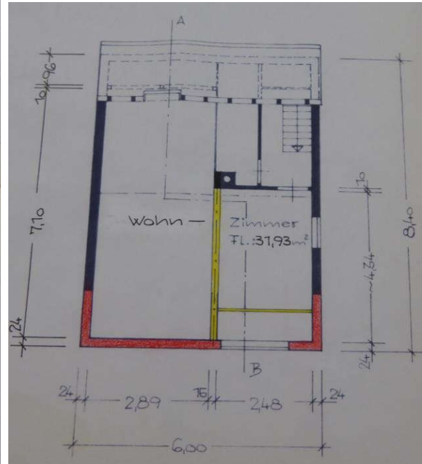
Grundriss DG Dachgeschossausbau 1974
