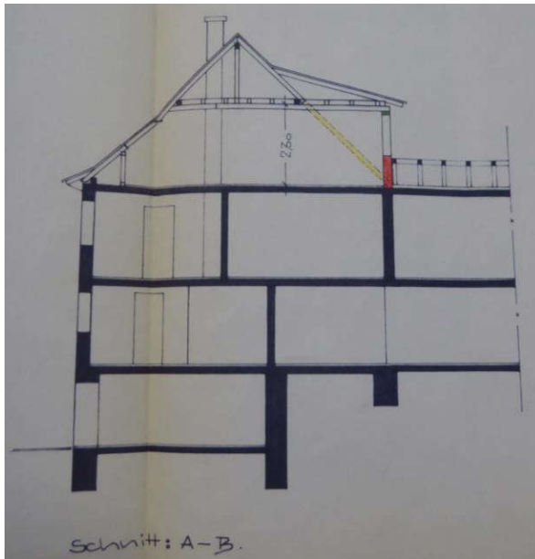
Schnitt DG-Ausbau aus 1974
