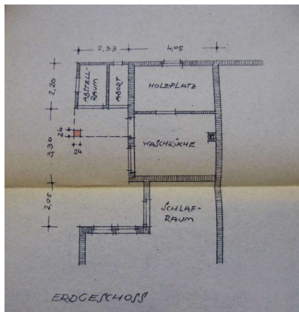
Grundriss EG Anbau 1961
