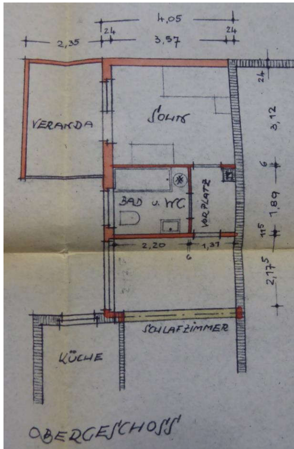
Grundriss OG Aufstockung Anbau 1961
