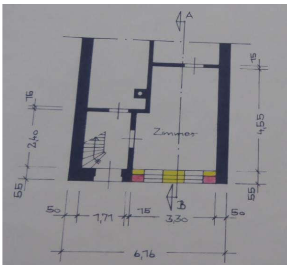
Grundriss EG Fassadenänderung 1973
