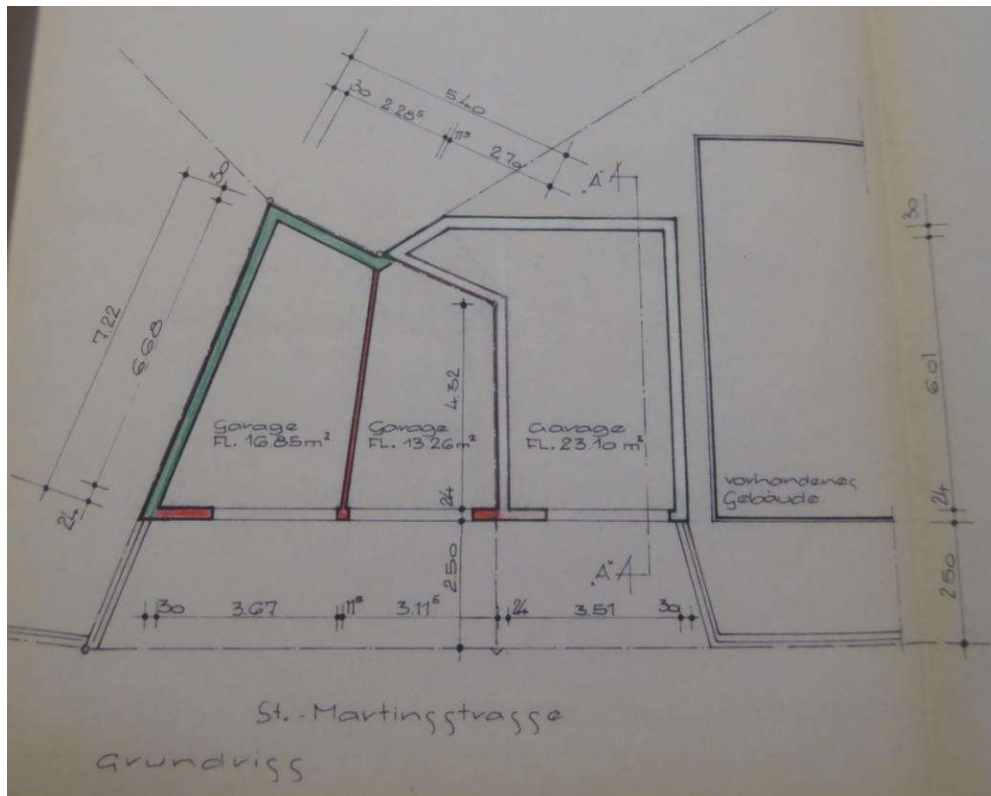
Grundriss Neubau Garagen 1968 (Bauantrag gemeinsam mit Garage auf Flst.Nr. 612/2)
