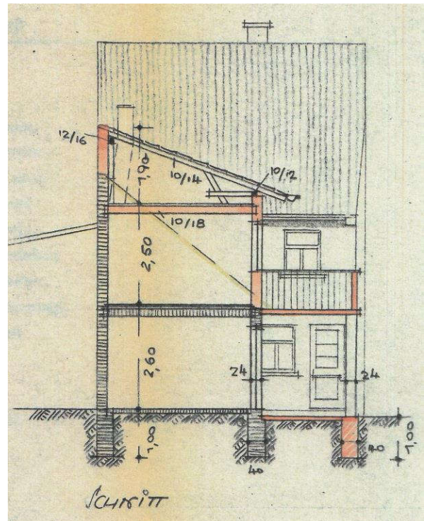
Schnitt Aufstockung Anbau 1961
