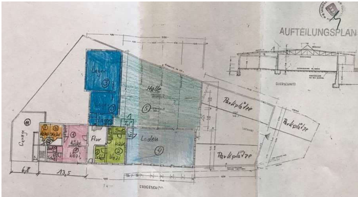
Abbildung 4 Erdgeschoss
