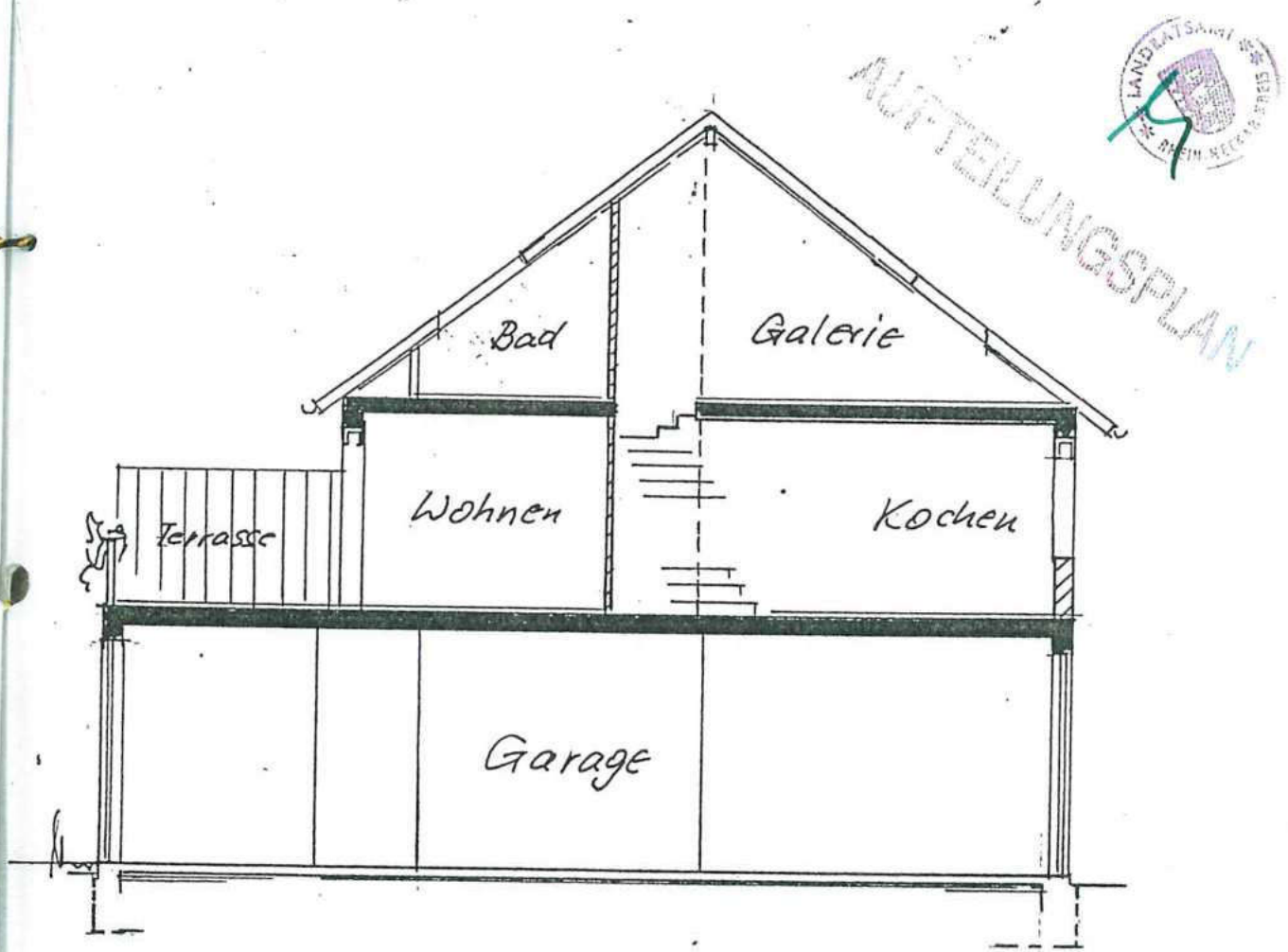
Schnitte A--A
