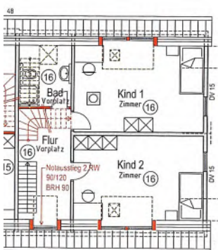
Dachgeschoss, Treppe nicht nutzbar
