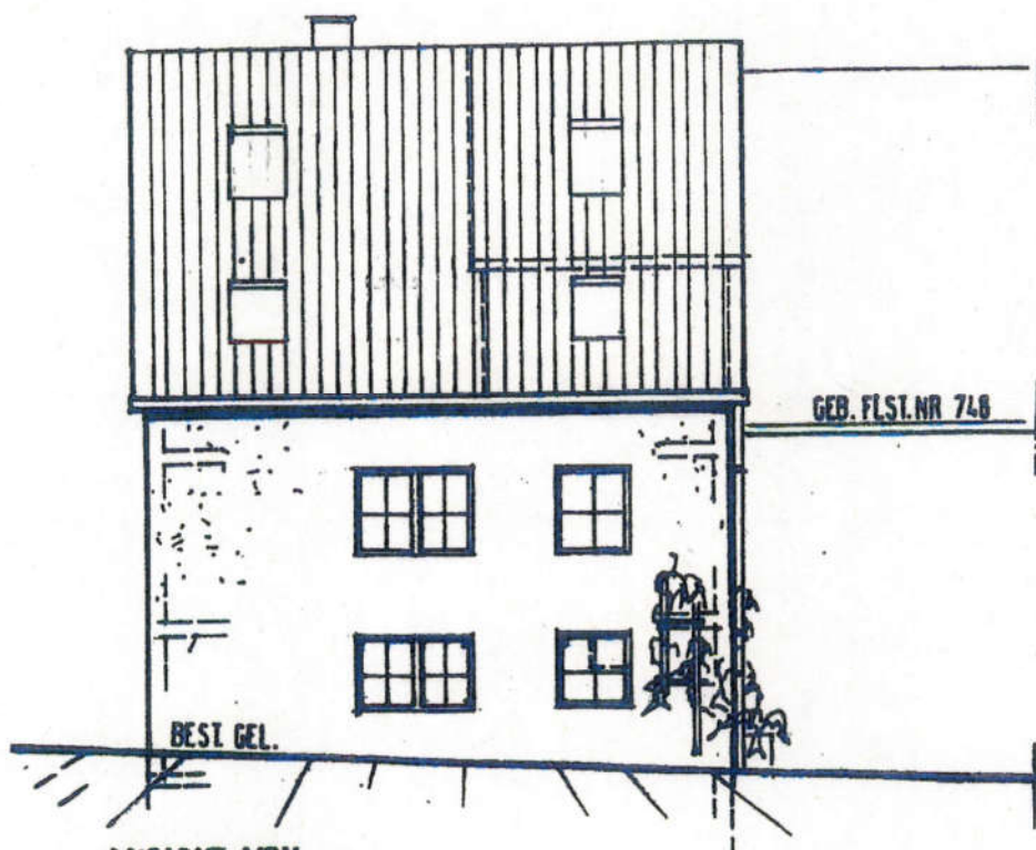
ANSICHT VON SÜD-WEST M. 1:100
