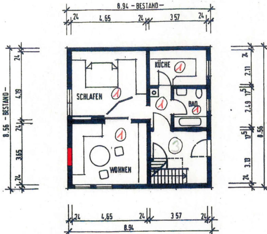
OBERGESCHOSS M 1:100
