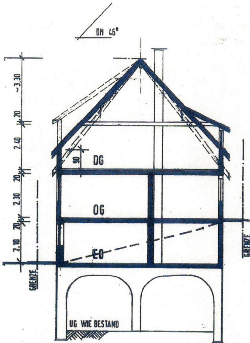
SCHNITT M 1:100
