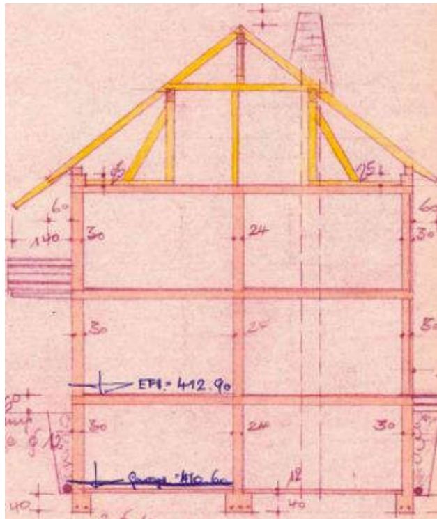
Schnitt
