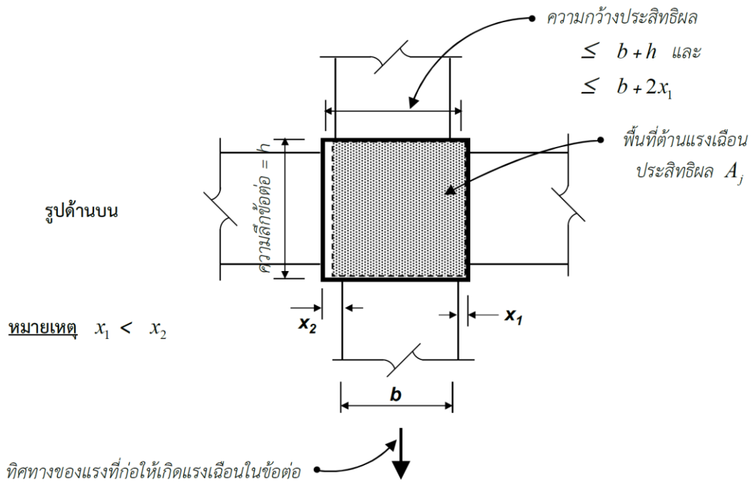
รูปที่ 5.2-7 พื้นที่ต้านแรงเฉือนประสิทธิภาพของข้อต่อระหว่างคานและเสา
