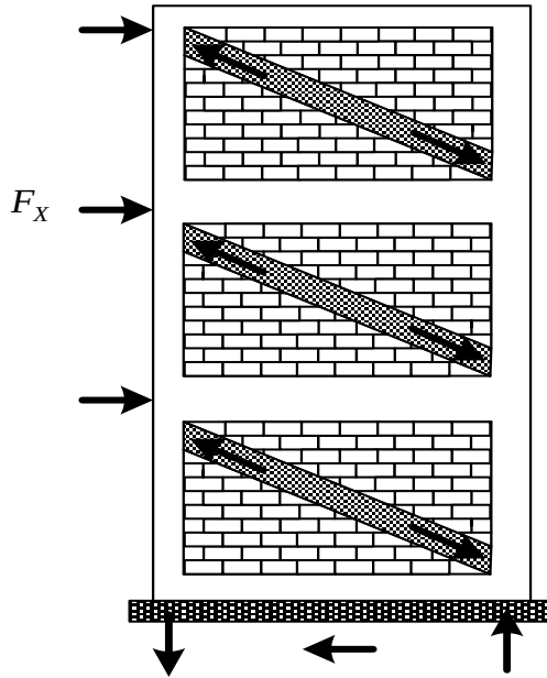
รูปที่ ง.3-2 ค้ำยันรับแรงอัดเทียบเท่า แบบเยื้องศูนย์
