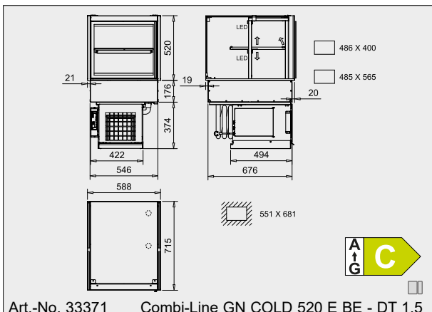
Art.-No. 33371 Combi-Line GN COLD 520 E BE - DT 1.5
