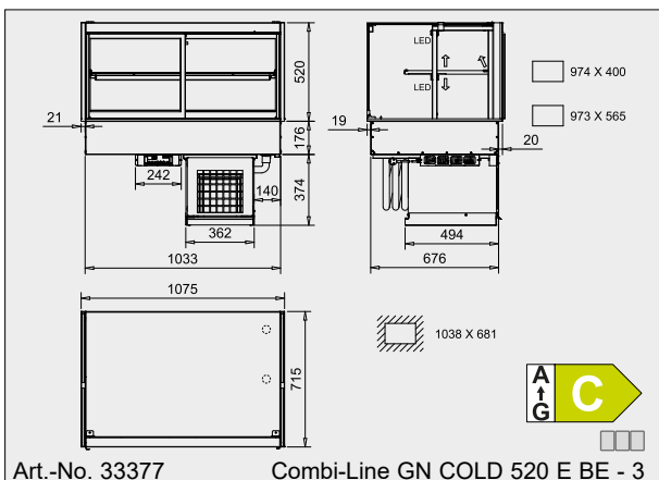
Art.-No. 33377 Combi-Line GN COLD 520 E BE - 3
