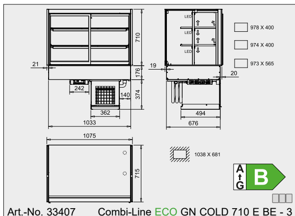
Art.-No. 33407 Combi-Line ECO GN COLD 710 E BE - 3
