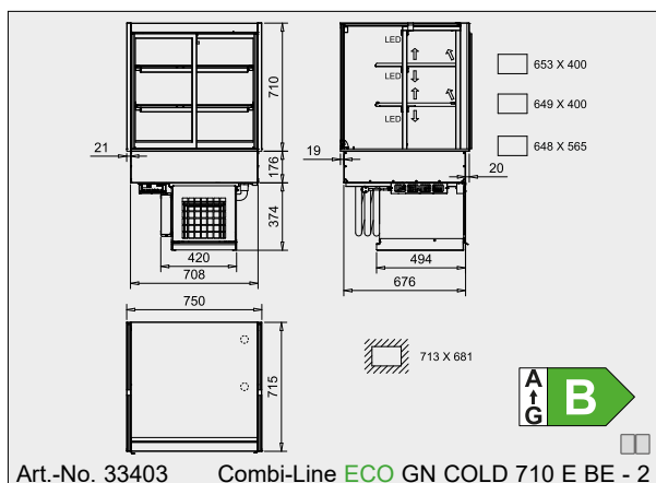
Art.-No. 33403 Combi-Line ECO GN COLD 710 E BE - 2
