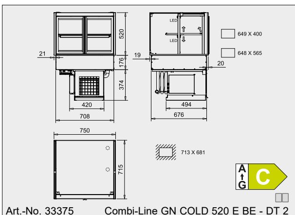
Art.-No. 33375 Combi-Line GN COLD 520 E BE - DT 2
