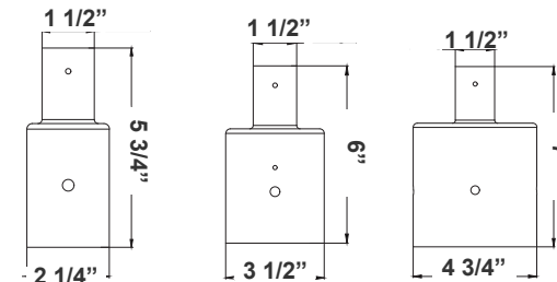
DAB-PA2-1 2 1/4"(W) x 5 3/4"(H) DAB-PA3-1 3 1/2"(W) x 6"(H) DAB-PA4-1 4 3/4"(W) x 7"(H)
