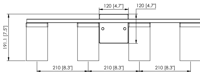
Technical Drawing: 7.5" (D) x 19.9" (W) x 7.1" (H)
