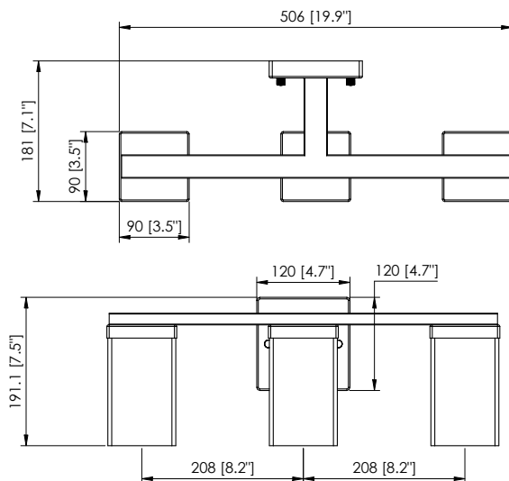
Technical Drawing: 7.5" (D) x 19.9" (W) x 7.1" (H)
