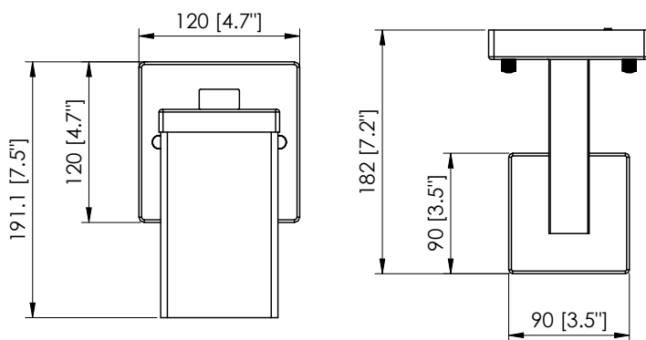
Technical Drawing: 3.5" (D) x 4.7" (W) x 7.5" (H)
