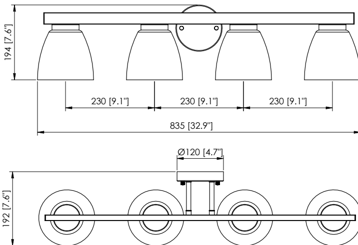
Technical Drawing: 7.6" (D) x 32.9" (W) x 7.6" (H)
