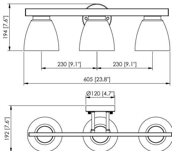
Technical Drawing: 7.6" (D) x 23.8" (W) x 7.6" (H)
