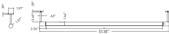
Technical Drawing: 1.97" (D) x 51.18" (W) x 5.79" (H)
