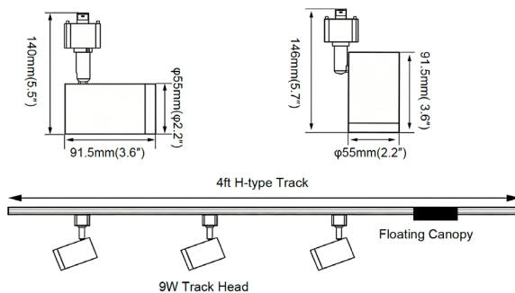
Technical Drawing: 5.5" (H) x 3.6" (W) x 2.2" (D)
