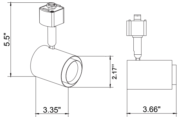
3.66" (W) x 5.5" (H) x 3.35" (D)
