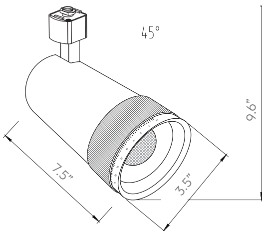
Technical Drawing: 7.5" (L) x 3.5" (D) x 9.6" (H)
