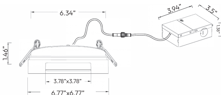
Technical Drawing: 6.77" (D) x 6.34" (W) x 1.46" (H)
