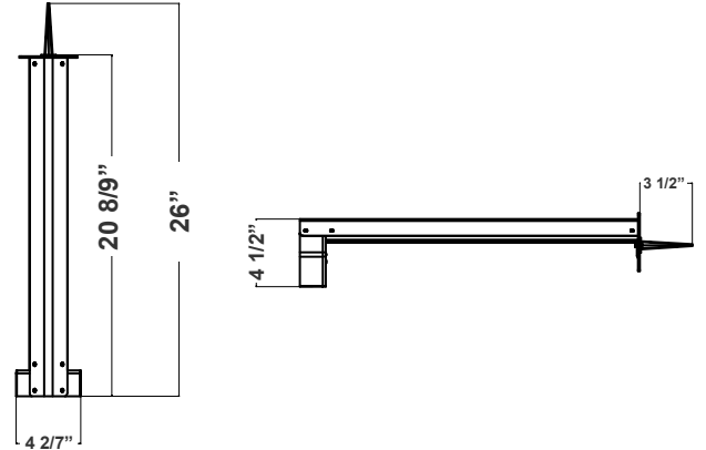
20 8/9"(H) X 4 2/7"(W) X 4 1/2"(D)
