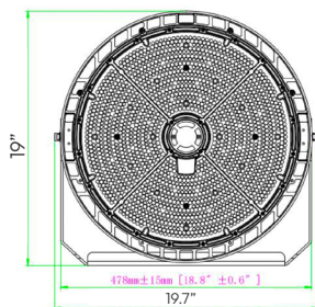
Technical Drawing: 19" (H) x 19.7" (W) x 22.9" (D)
