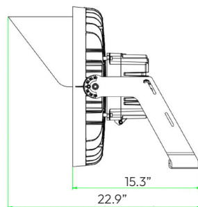
Technical Drawing: 19" (H) x 19.7" (W) x 22.9" (D)
