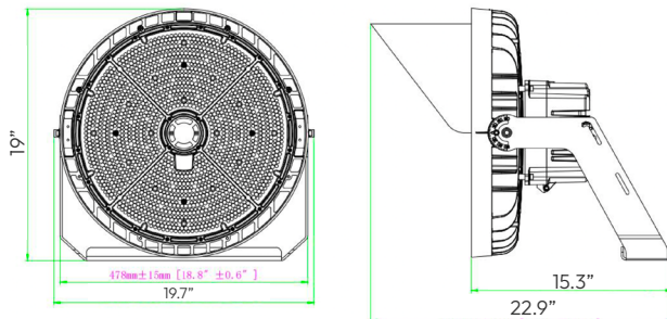
Technical Drawing: 19" (H) x 19.7" (W) x 22.9" (D)
