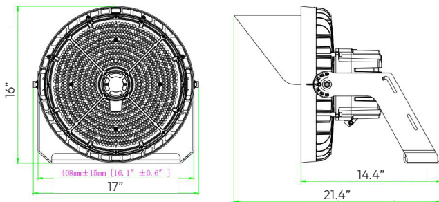
Technical Drawing: 16" (H) x 17" (W) x 21.4" (D)
