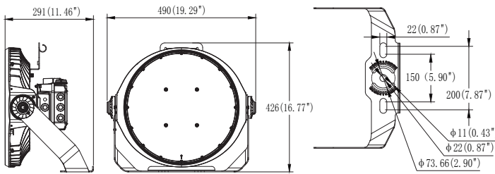
Technical Drawing: 11.46" (D) x 19.29" (W) x 16.77" (H)
