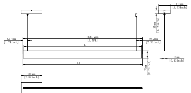
SCSSL-UD-8FT-MCTP SCSSL-REC 3.7"(W) x 2.76"(H) x 4.33"(D)
